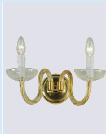
Art. 345/ A2 L 35 cm H 28 cm (in. 13,75x11,00) 2 x 40W E14 Peso/Weight Kg. 3 (Lb 6,62)
